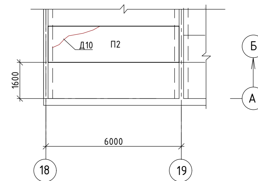
Схема расположения дефекта плиты П2 между осями 18-19/А-Б
