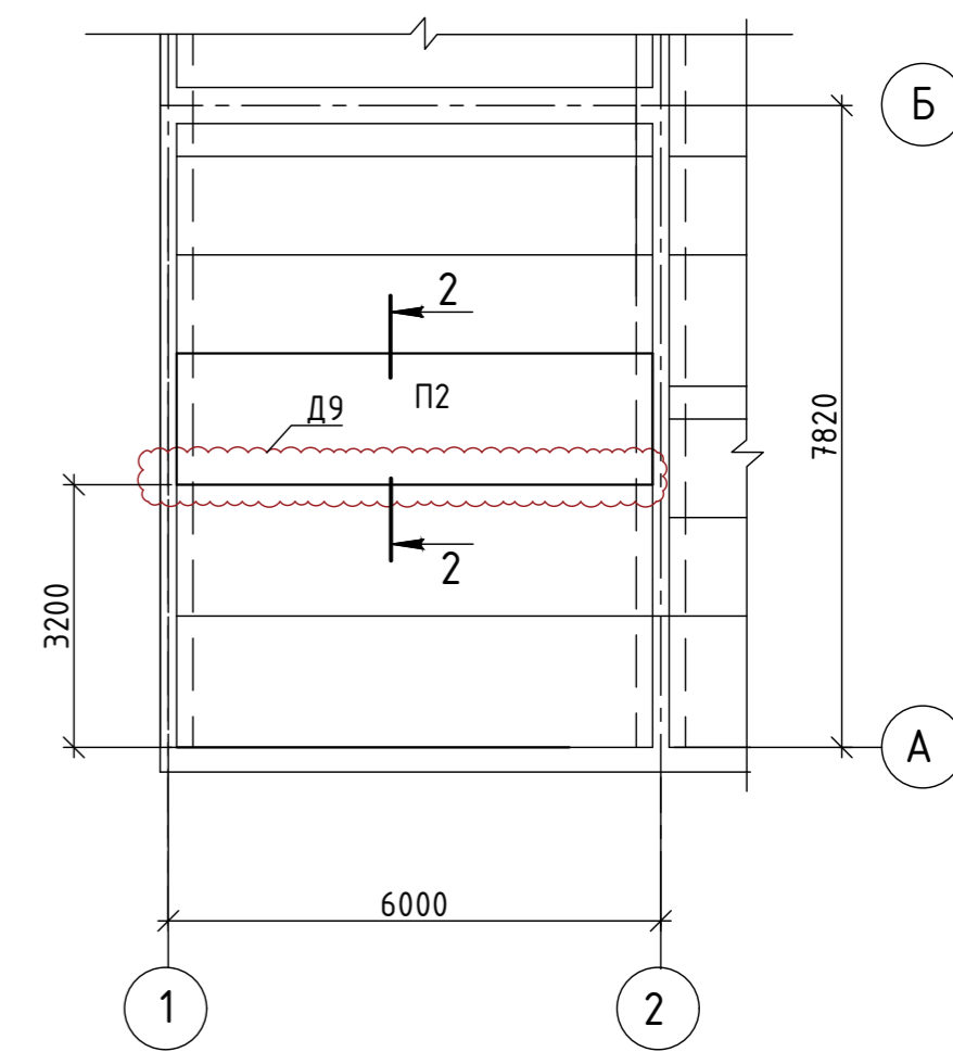
Схема расположения дефектов плиты П2 между осями 1-2/А-Б
