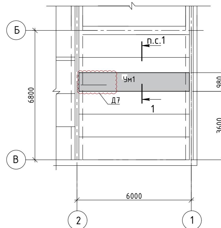
Схема расположения дефектов монолитного участка Ум1 между осями 2-1/В-Б
