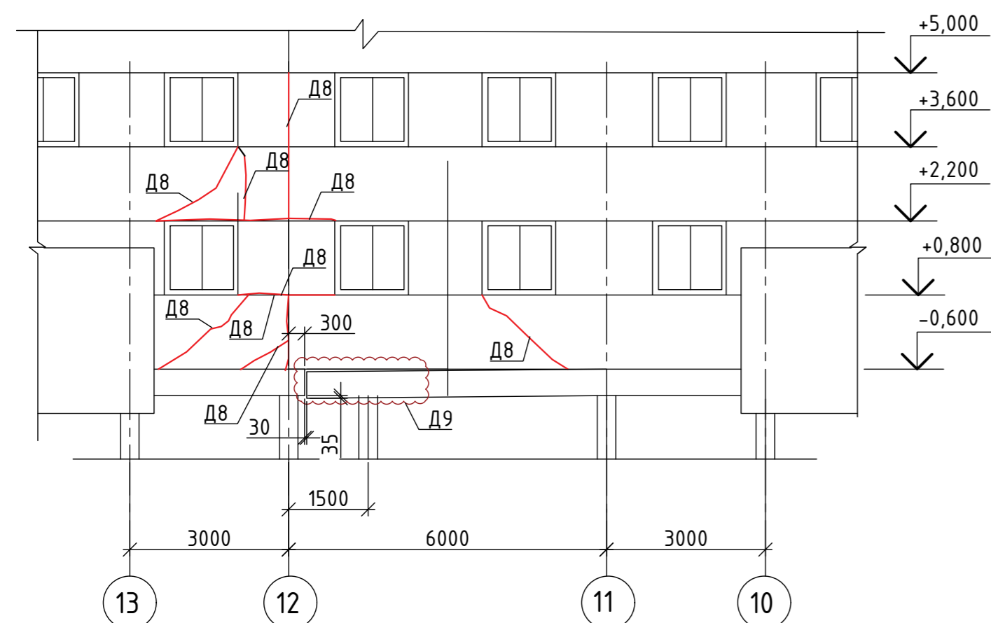
Схема расположения дефектов наружных стен между осями 13-12/В-Б
