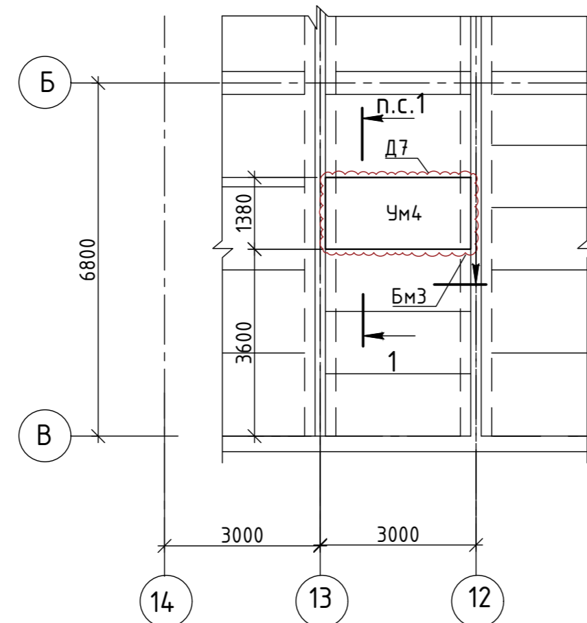
Схема расположения дефектов монолитного участка Ум4 между осями 13-12/В-Б
