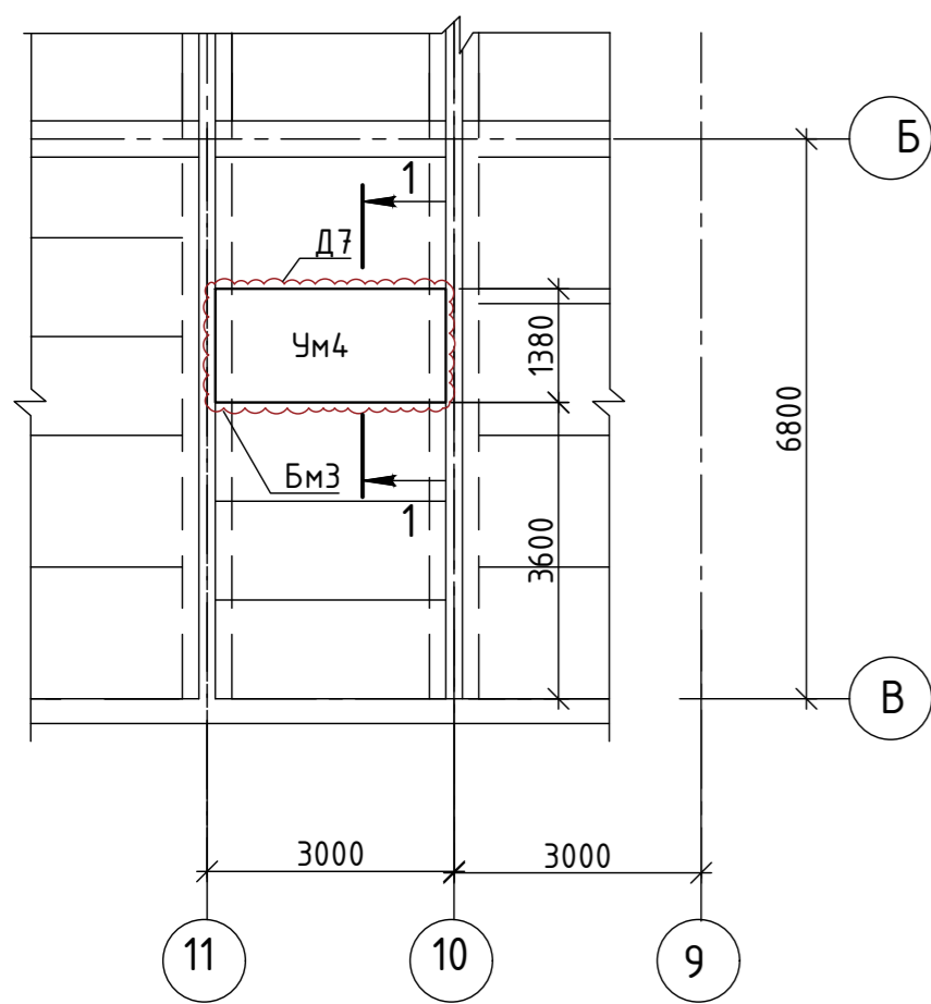
Схема расположения дефектов монолитного участка Ум4 между осями 11-10/В-Б
